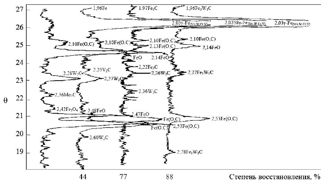
Рис. 2. Фрагменты дифрактограмм проб окалины стали P6M5 с разной степенью восстановления. Цифры возле кривых отвечают степени восстановления
