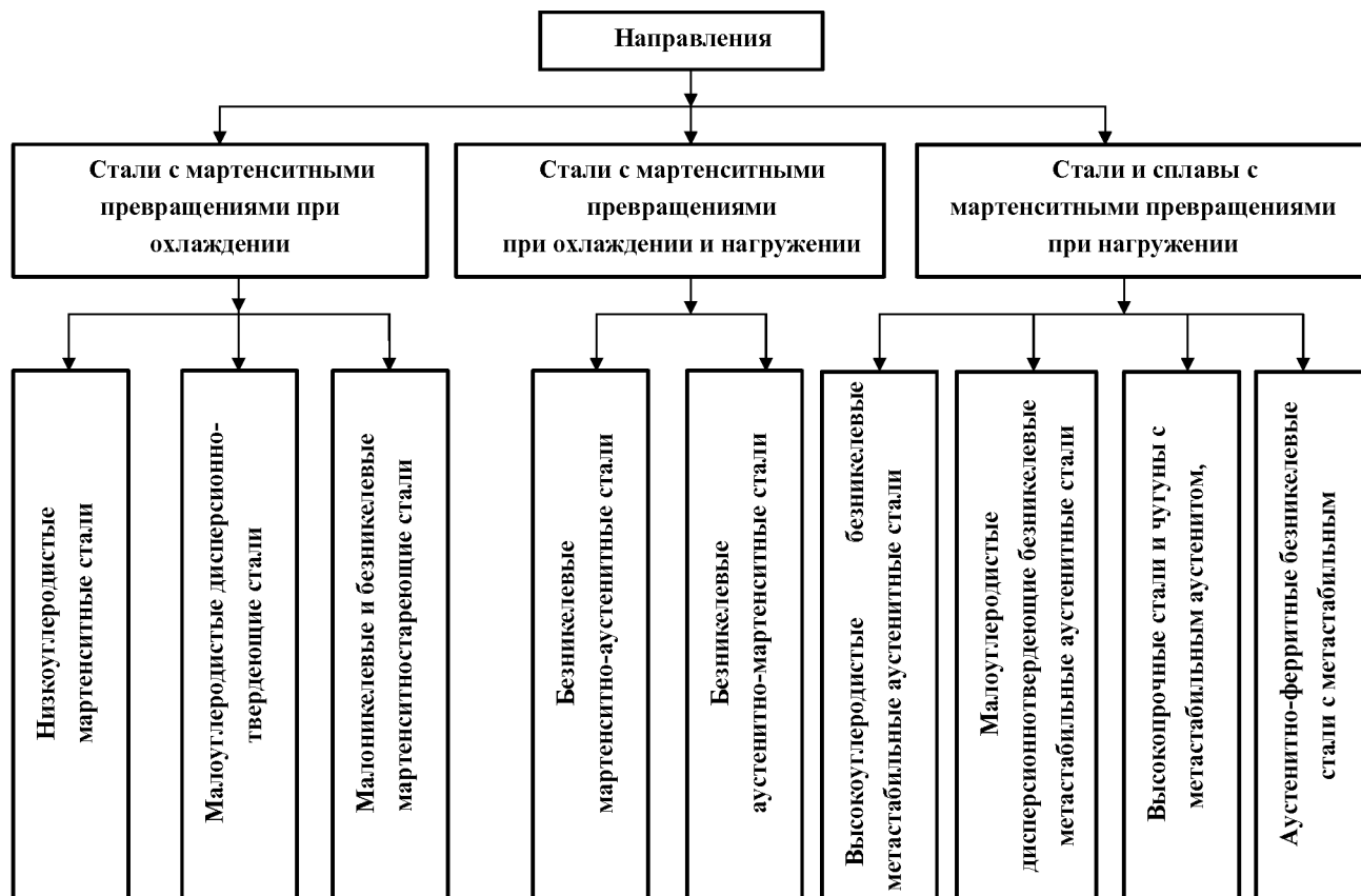
Рис. 1. Перспективные направления в создании экономнолегированных высокопрочных сталей
