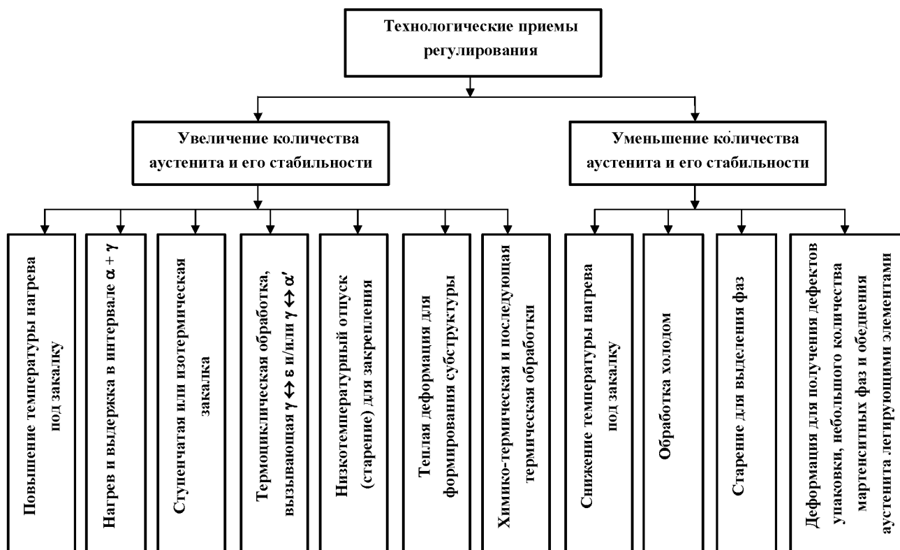
Рис. 3. Технологические приемы регулирования количества и устойчивости аустенита
