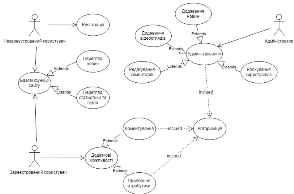
Рисунок 3.4 - Діаграма прецедентів програмного забезпечення для надання інформації про спортивні клуби у нотації UML
