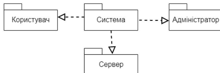
Рисунок 3.2 - Діаграма пакетів програмного забезпечення для надання інформації про спортивні клуби у нотації UML
