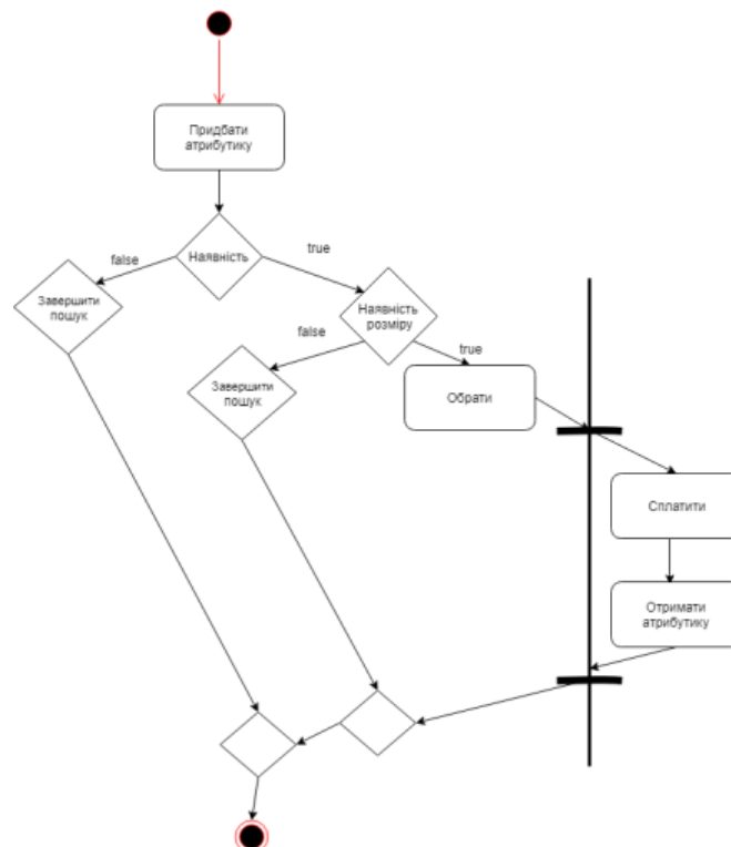
Рисунок 3.5 - Діаграма діяльності програмного забезпечення для надання інформації про спортивні клуби у нотації UML
