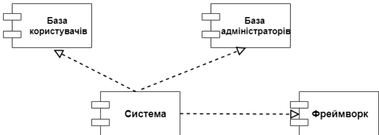
Рисунок 3.3 - Діаграма компонентів програмного забезпечення для надання інформації про спортивні клуби у нотації UML
