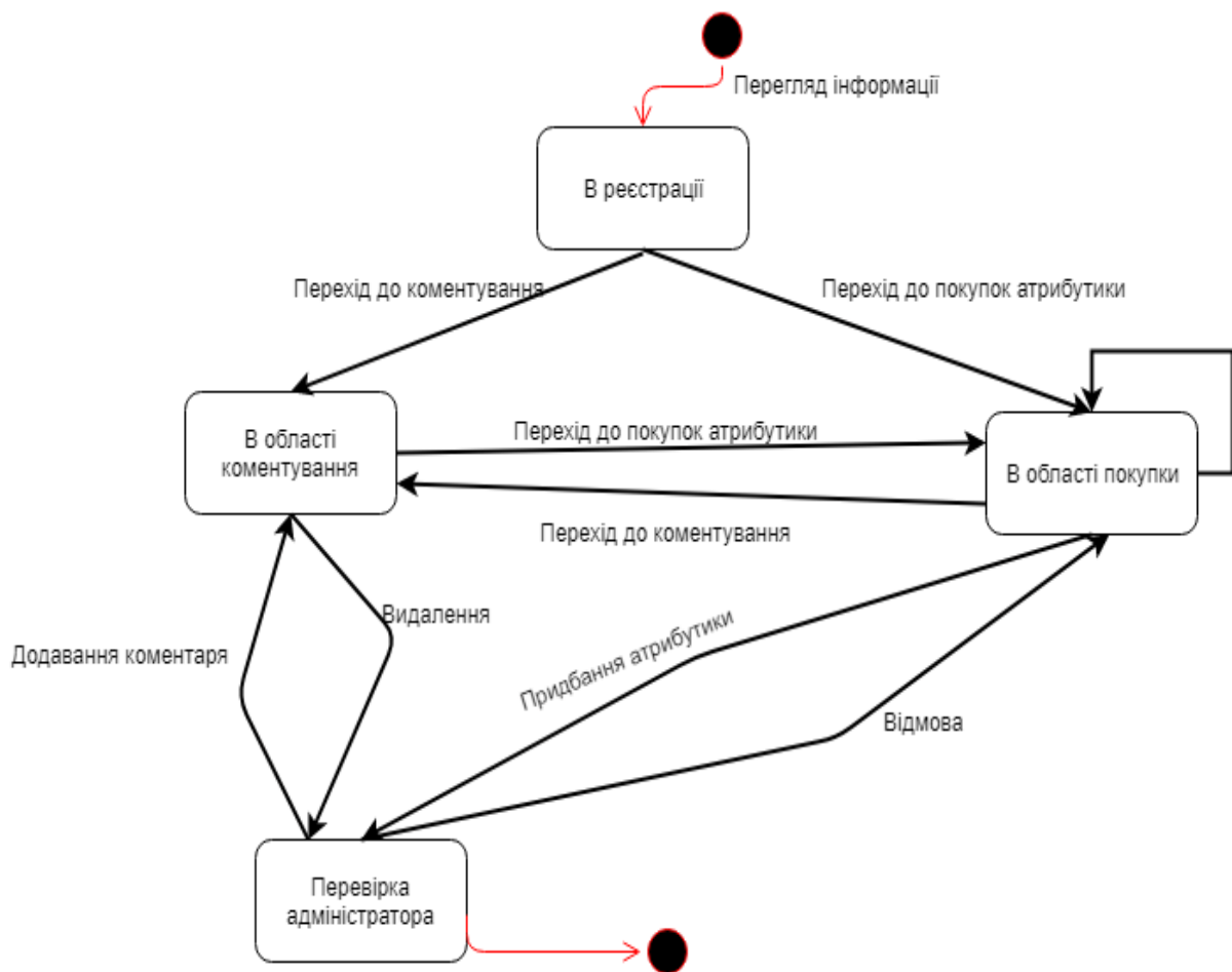
Рисунок 3.6 - Діаграма станів програмного забезпечення для надання інформації про спортивні клуби у нотації UML
