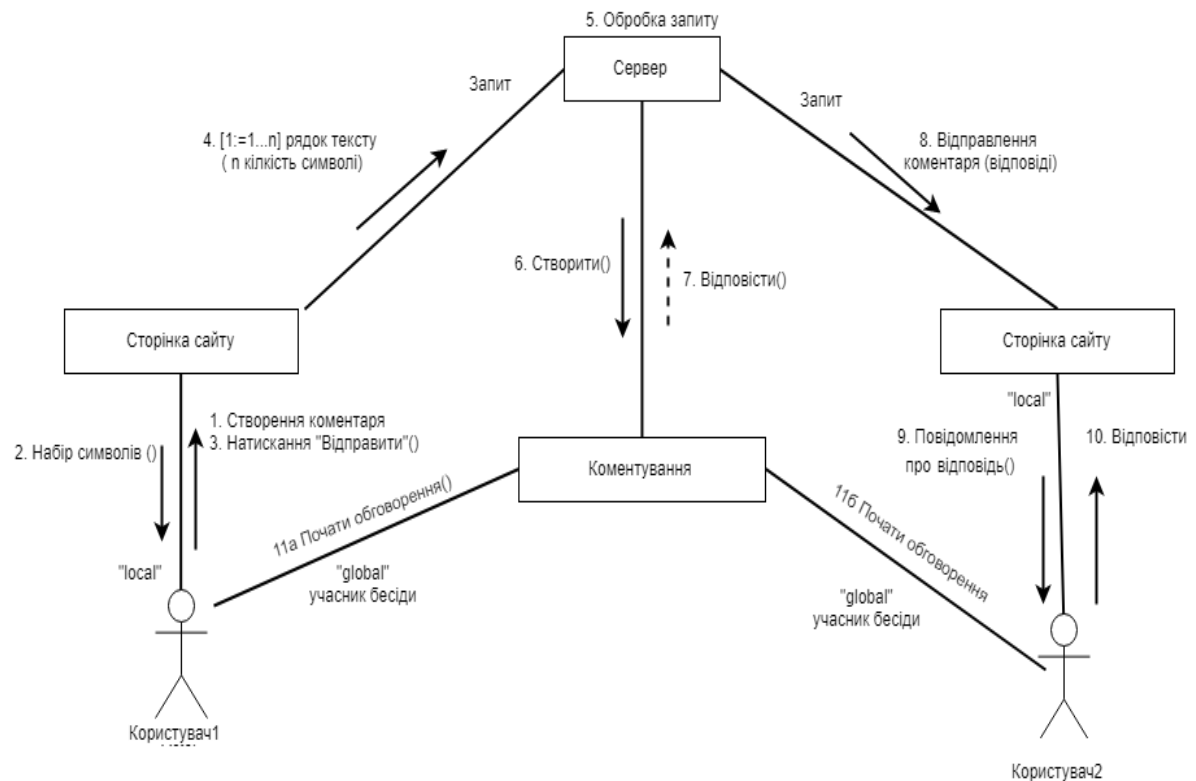
Рисунок 3.8 - Діаграма кооперацій програмного забезпечення для надання інформації про спортивні клуби у нотації UML
