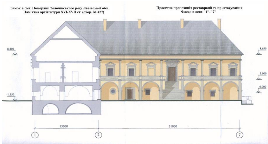
Рисунок 2.1 – Фасад замку в Поморянах
