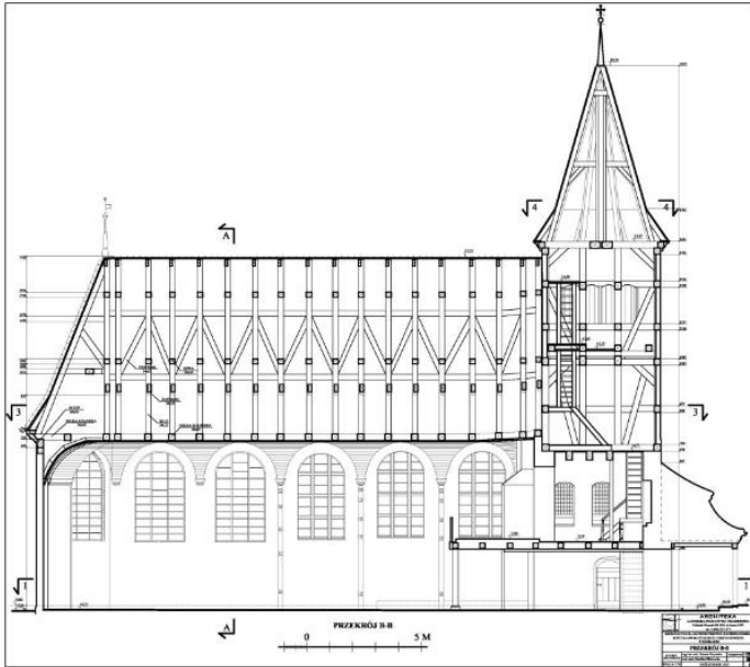
Рисунок 2.3 – Перетин храму із показом конструктивних рішень
