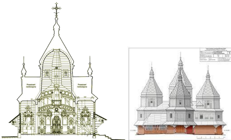
Рисунок 5.2 – Обміри церкви. Переріз
