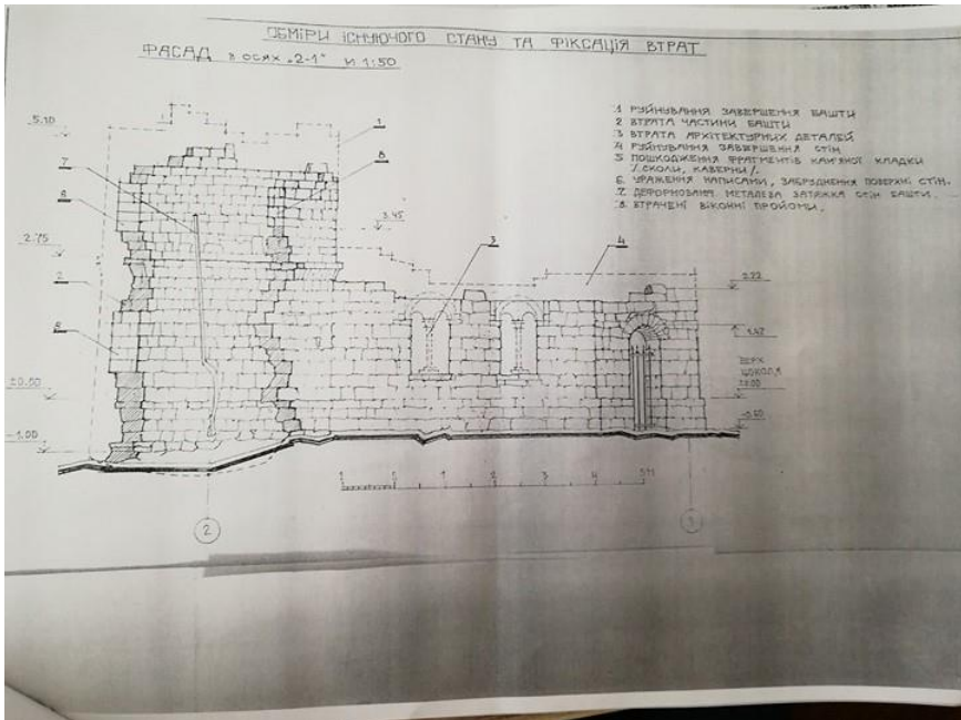
Рисунок 5.1 – Обміри баштової стіни
