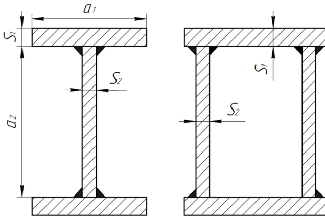
а – двотавровий переріз; б – коробчастий переріз
