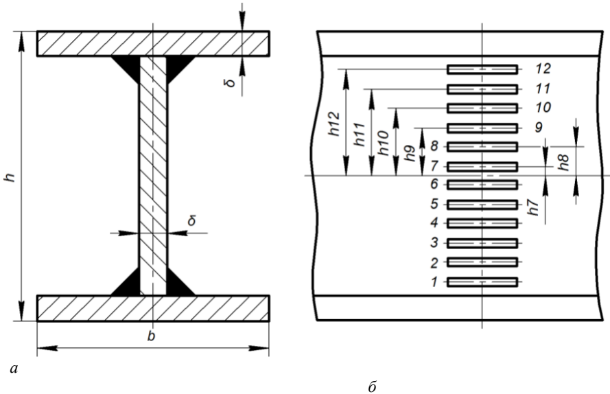
a – переріз балки; b – 1...12 – номери тензорезисторів (перерізів)
