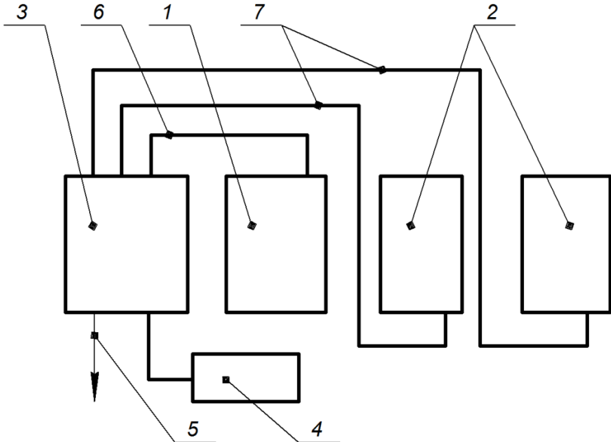
Рисунок 4.3 – Блок-схема приладу ЦТК-1
