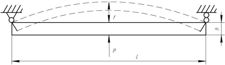
Рисунок 2.3 – Схема прикладення навантаження на двоопорну балку Дослідження розподілення напружень в балці виконаємо розрахунковим та експериментальним шляхом.
