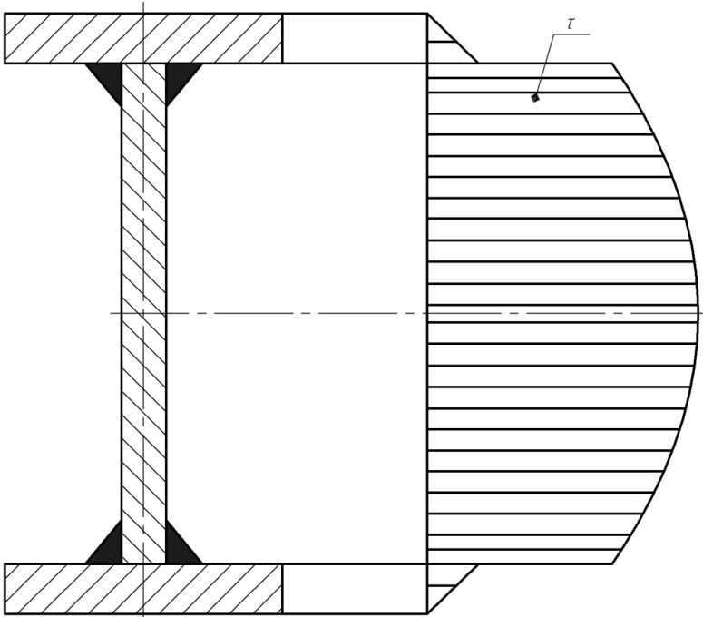
Рисунок 2.5 – Розподіл (епюра) дотичних напружень \tau по висоті балки
