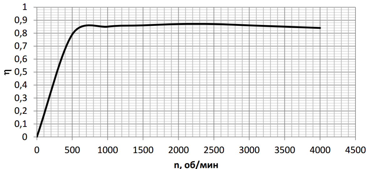
Рис. 1. Залежність ККД тягового двигуна від швидкості обертання вала двигуна
