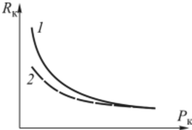
Рисунок 1.3 – Залежність перехідного контактного опору від сили контактного натиску
