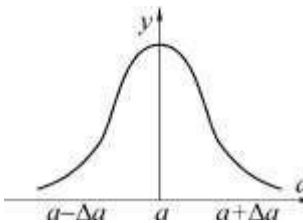
Рисунок А.1 – Крива Гауса
