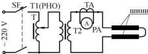
Рисунок 2.1 – Схема дослідження ЕДЗ плоских шин.
