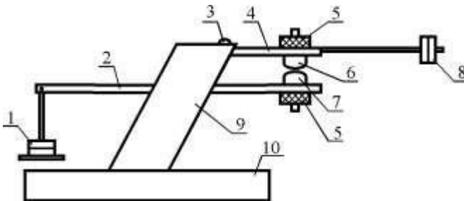
Рисунок 1.4 – Ескіз експериментальної установки.
