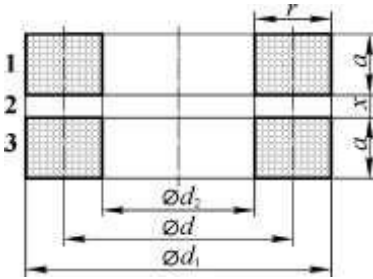
Рисунок Б.1 – До визначення взаємної індуктивності котушок
