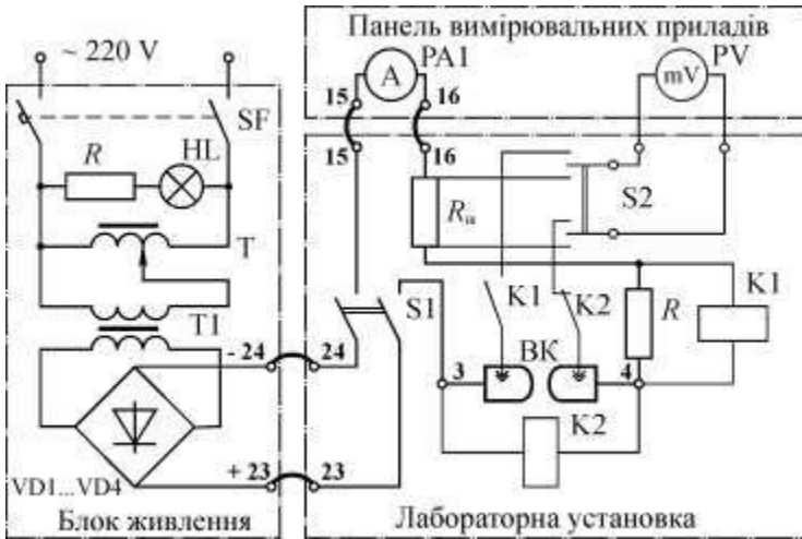
Рисунок 1.5 – Електрична схема установки.
