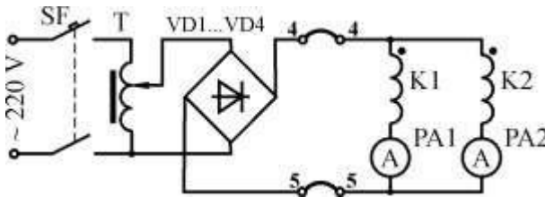
Рисунок 2.2 – Схема дослідження ЕДЗ кругових кілець (котушок)
