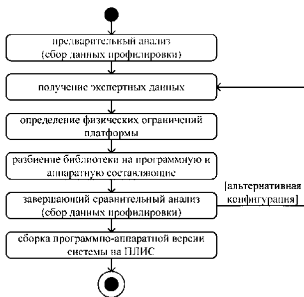
Рис. 2. Методика разработки системы на ПЛИС, использующей программно-аппаратную реализацию математической библиотеки
