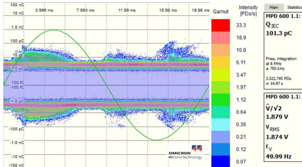
Рисунок 2.1 – Приклад АФД масла наповненого трансформатору струму з частковими розрядами в ізоляції
