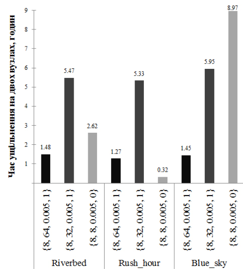
Рисунок 6 – Час ущільнення на 2х вузлах
