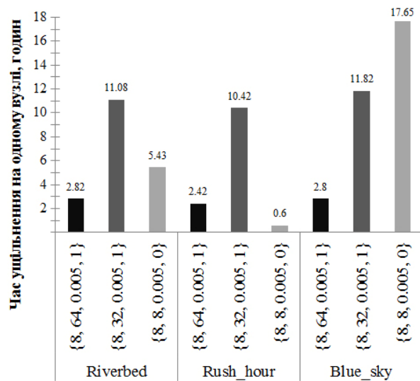
Рисунок 5 – Час ущільнення на одному вузлі
