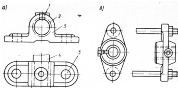
Рисунок 5.2 – Підшипники з суцільним корпусом
