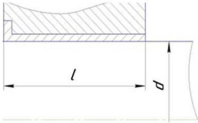
Рисунок 5.1 – Конструкція вкладня.
