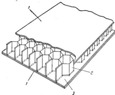
Рисунок 3.1 - Панель стільникової конструкції
