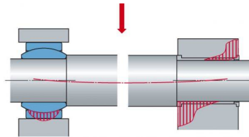
Рисунок 5.6 – Приклади закріплення вала у підшипниках
