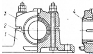
Рисунок 5.3 – Підшипник з рознімним корпусом
