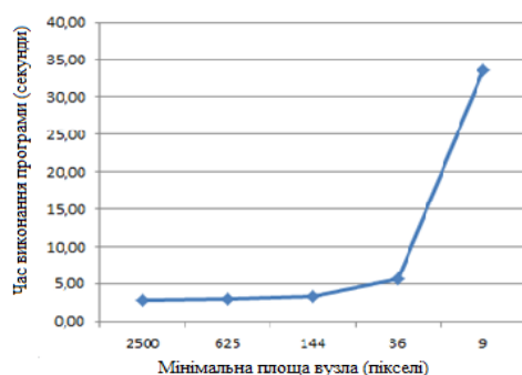
Рисунок 4 – Залежність часу роботи програми від площі вузла
