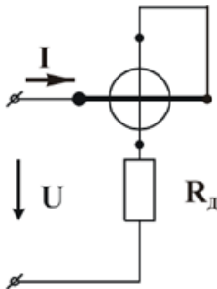
Рисунок 4.18 – Вольтметри електродинамічної системи
