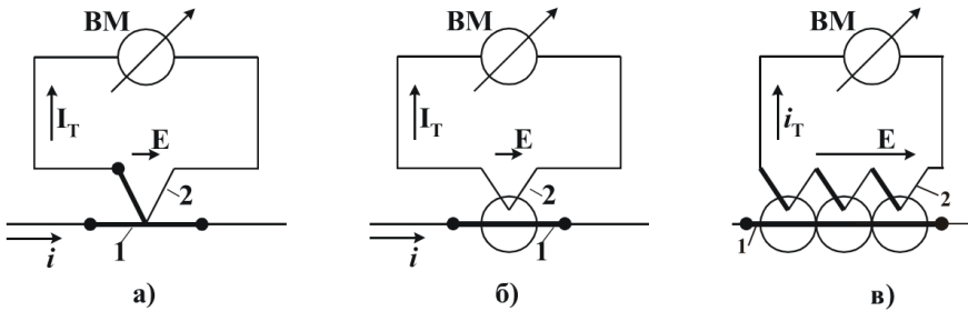
Рисунок 4.13 – Схеми підключення термоперетворювача
