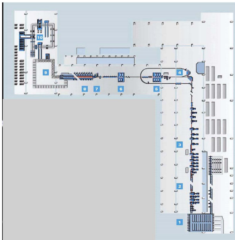
Рис. 8. Проволочный прокатный стан в Дуйсбурге:
