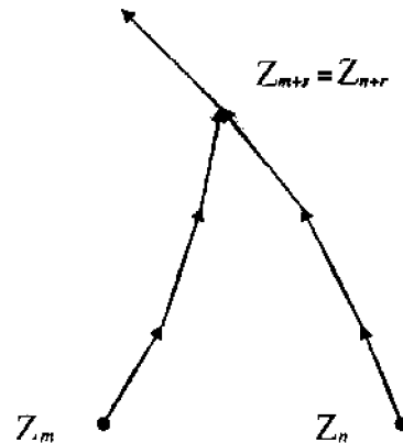
Рис. 2. \lambda -метод Полларда
