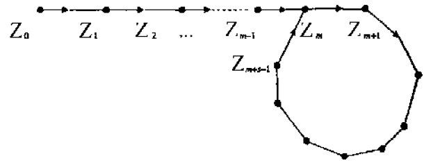
Рис. 1. \rho -метод Полларда
