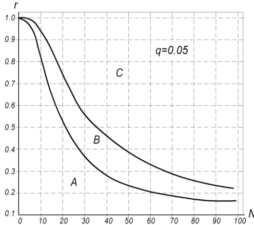
Рисунок 3.2 – Графік для визначення значимості коефіцієнта кореляції
