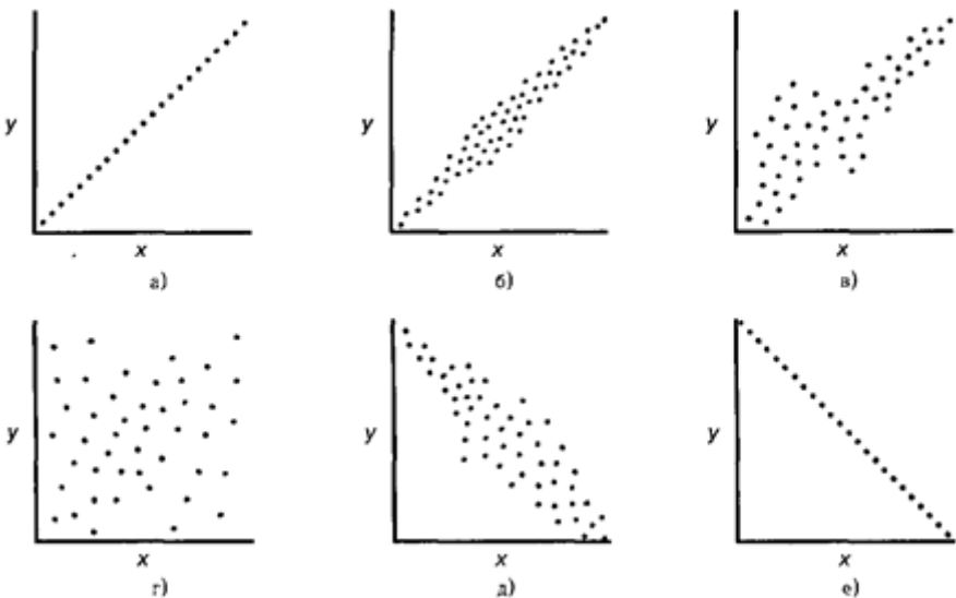
а, б, в, д, е – зв'язок існує; г – зв'язку немає Рисунок 3.1 – Визначення наявності кореляційного зв'язку.
