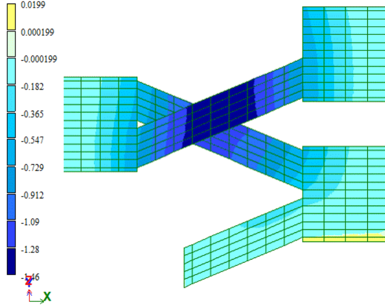
Рисунок 18-ізополя переміщень по осі Z по 2 навантаженню (РПН 2)
