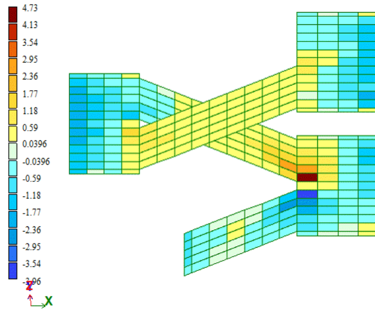
Рисунок 29- Мозаика напряжень по M_y згідно РПЗ
