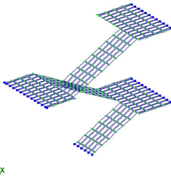
Рисунок 6- Розрахункова модель в просторі ПК ЛИРА-САПР
