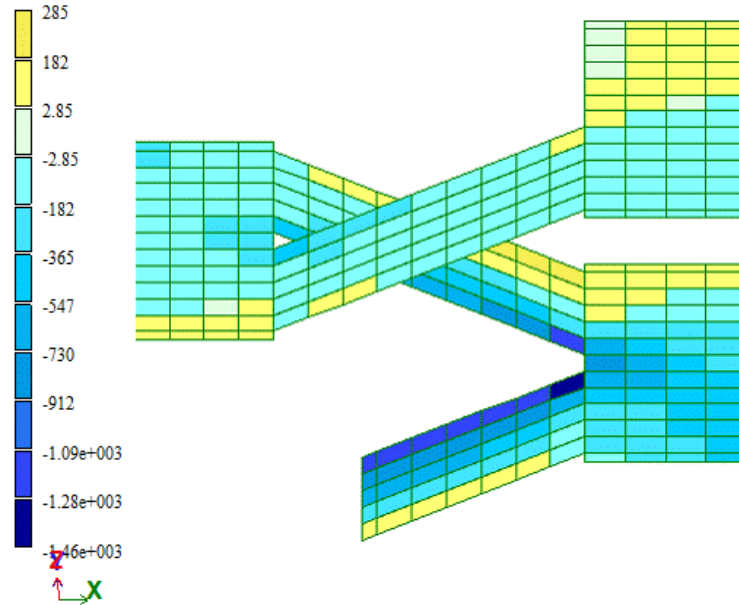
Рисунок 26-Мозаика напряжень по N_x згідно РПН
