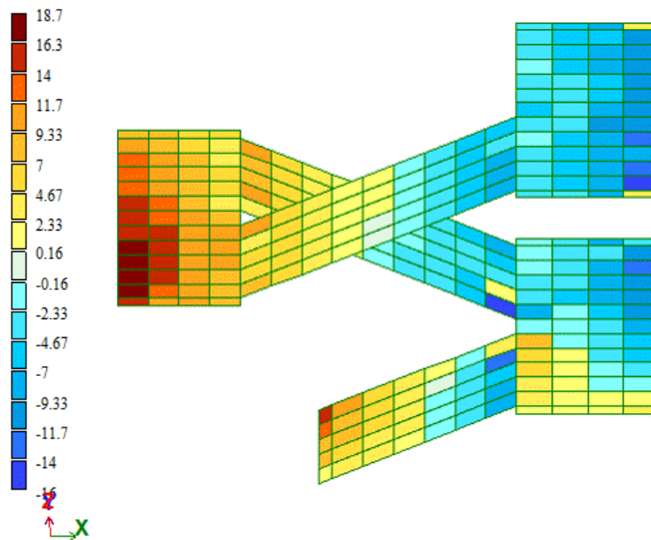
Рисунок 30-Мозайка напряжень по Q_x згідно РПЗ
