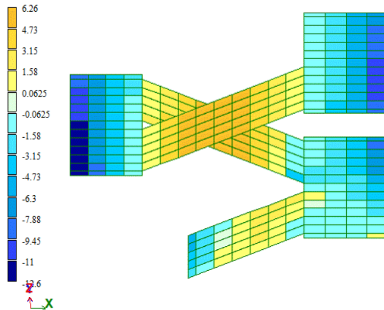
Рисунок 22- Мозаика напряжень по M_x згідно РПН
