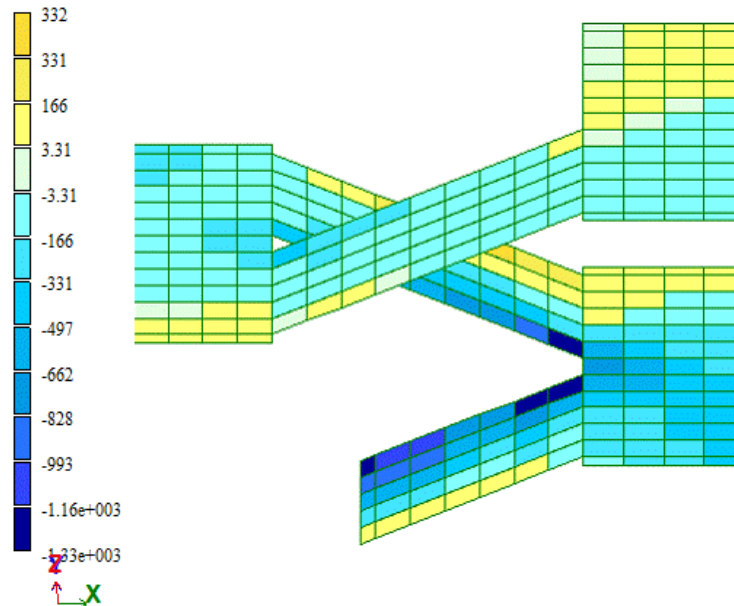
Рисунок 32-Мозаика напряжень по N_x згідно РПЗ
