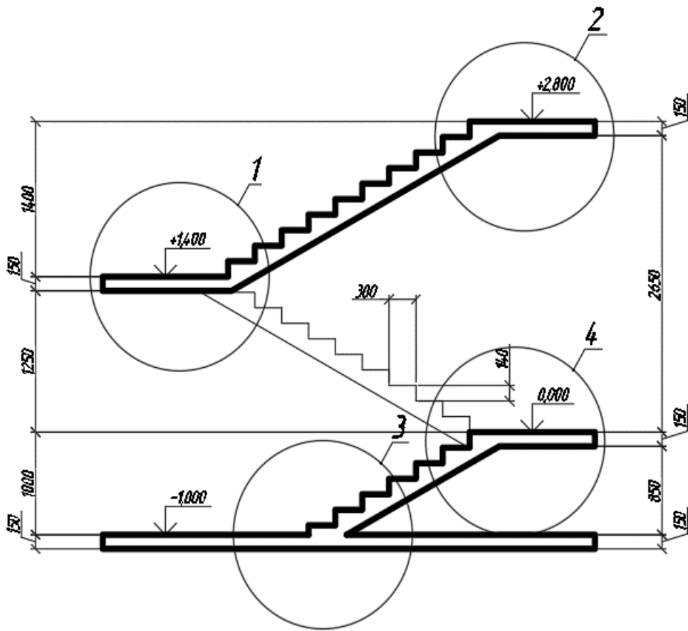
Рисунок 1- Схема сходової клітини.
