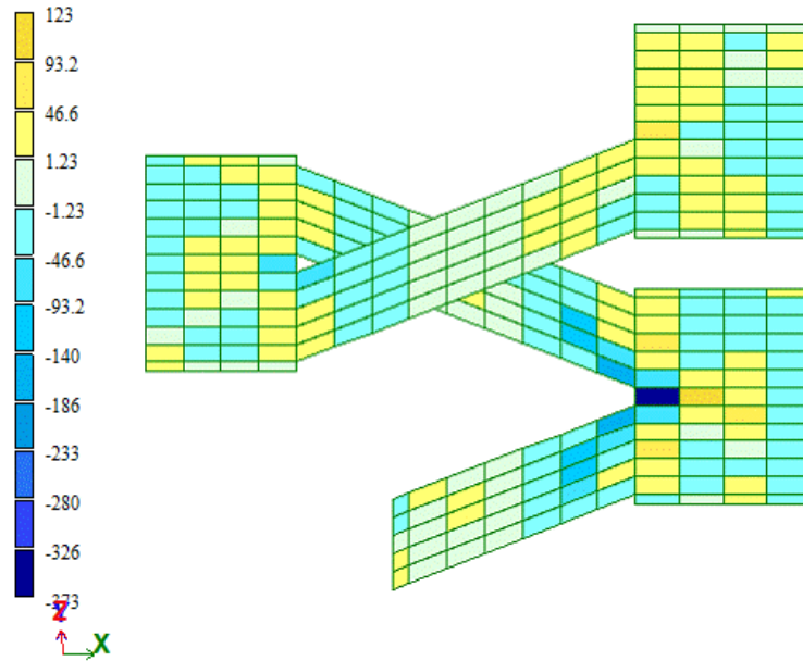
Рисунок 33-Мозаика напряжень по N_y згідно РПЗ
