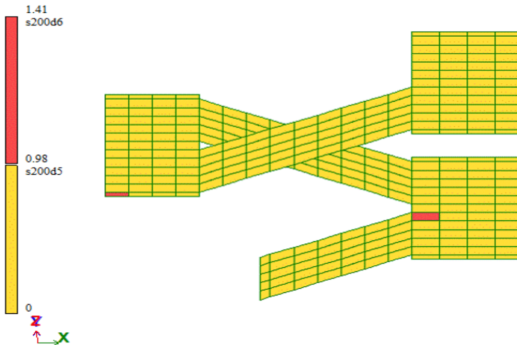
Рисунок 34- Плоца верхньої арматури по осі Y
