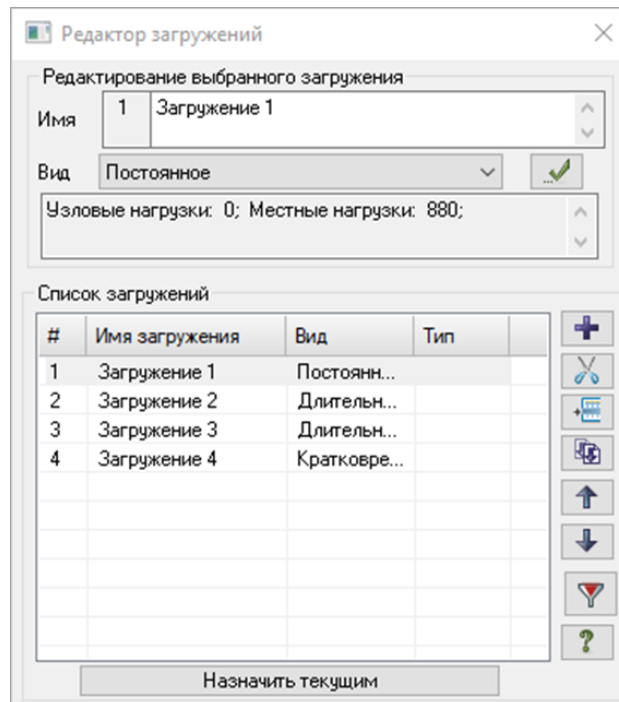
Рисунок 5- Встановлення навантажень та їх характеристика
