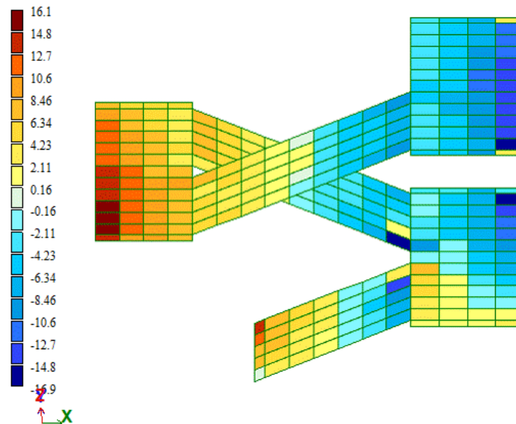
Рисунок 24-Мозайка напряжень по Q_x згідно РПН
