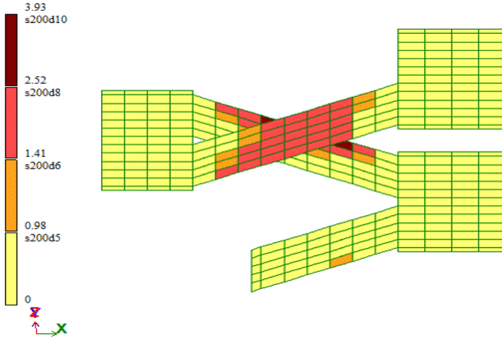
Рисунок 37- Площа нижньої арматури по осі X
