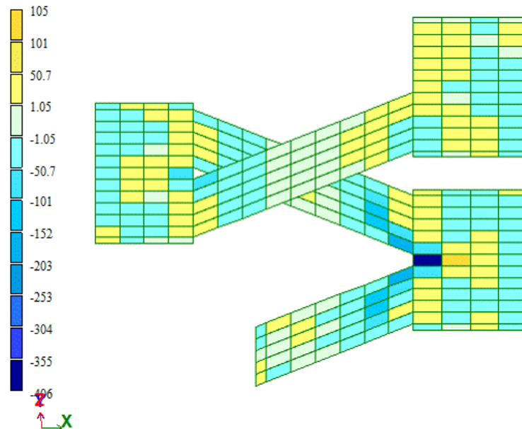
Рисунок 27-Мозаика напряжень по N_y згідно РПН
