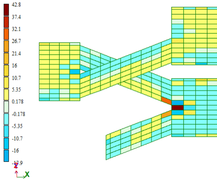
Рисунок 31-Мозайка напряжень по Q_y згідно РПЗ
