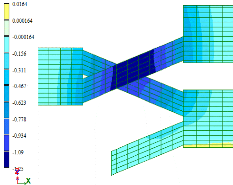
Рисунок 19-Ізополя переміщень по осі Z по 3 навантаженню (РПН 3)
