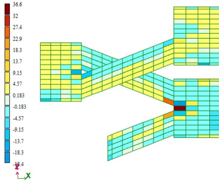
Рисунок 25-Мозайка напряжень по Q_y згідно РПН
