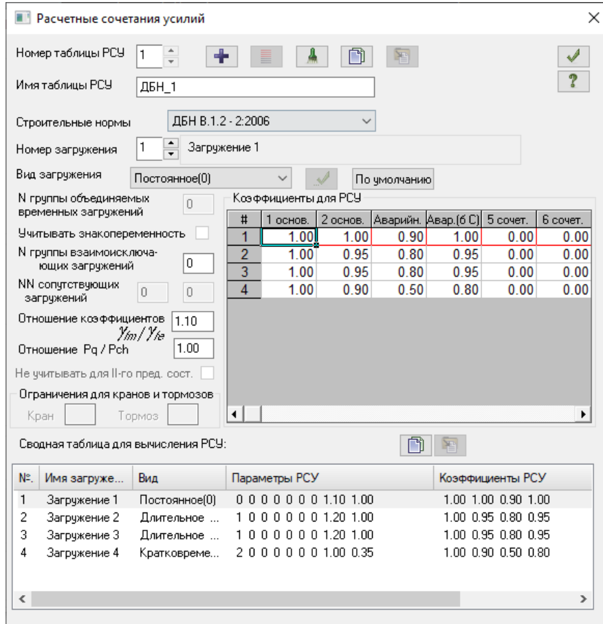
Рисунок 15- Таблица розрахункових поєднань зусиль.
