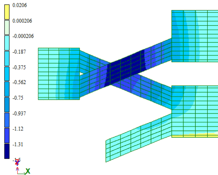
Рисунок 17-Изополя переміщень по осі Z по 1 навантаженню (РПН 1)
