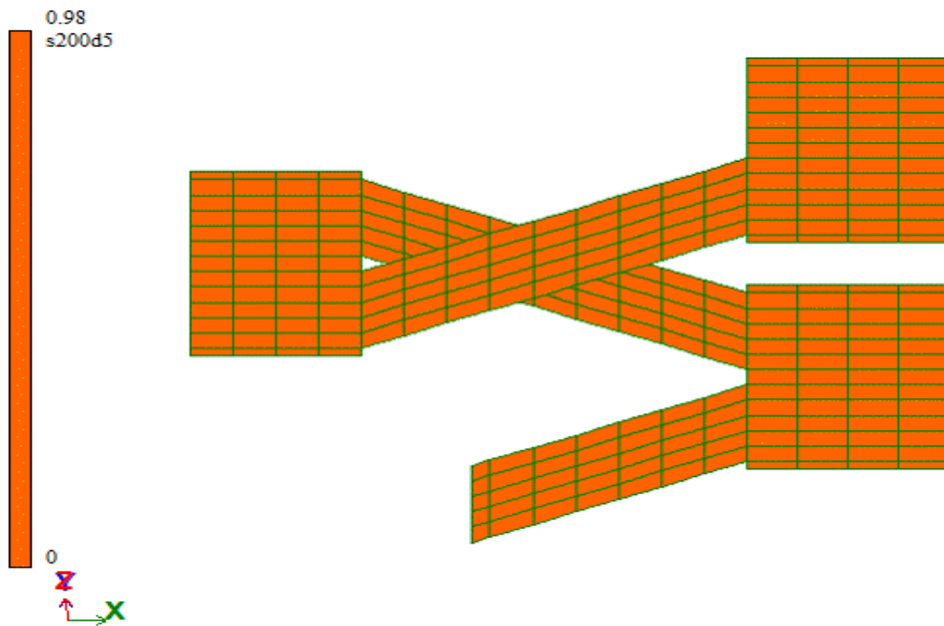
Рисунок 36- Площа нижньої арматури по осі Y
