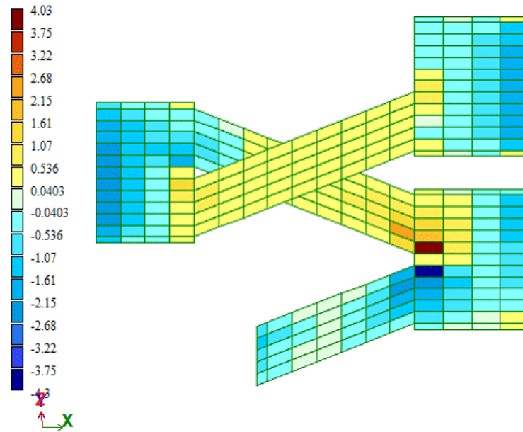
Рисунок 23- Мозаика напряжень по M_y згідно РПН
