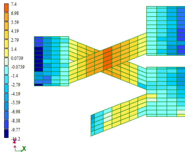
Рисунок 28- Мозаика напряжень по M_x згідно РПЗ
