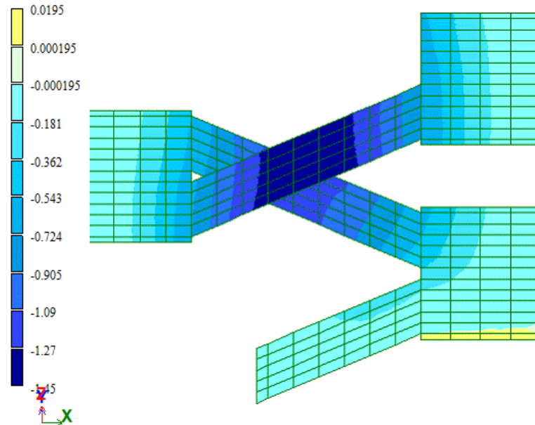
Рисунок 20 Ізополя переміщень по осі Z по 4 навантаженню (РПН 4)
